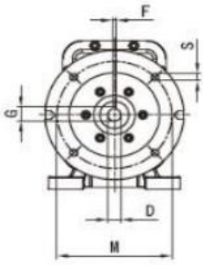
Wymiary kołnierza PAM
