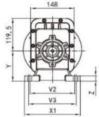
Wymiary łań przekładni DRC03
