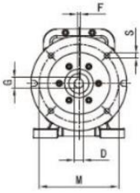
Wymiary kołnierza PAM
