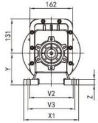
Wymiary łap przekładni DRC04
